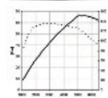
----- Teljesítmény ----- Forgatónyomaték
